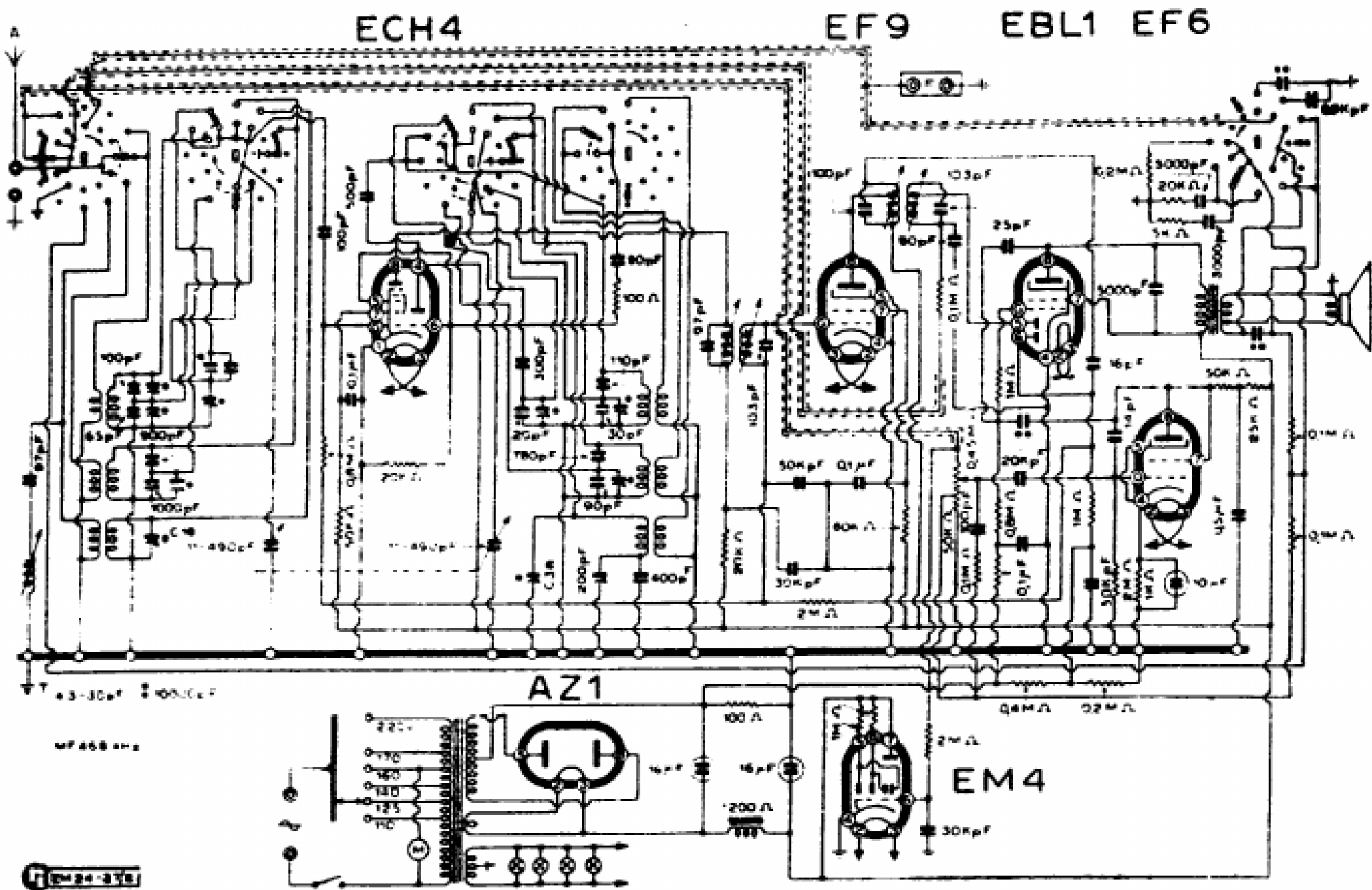
PHILIPS RADIO - MOD. « DI 580/A »
